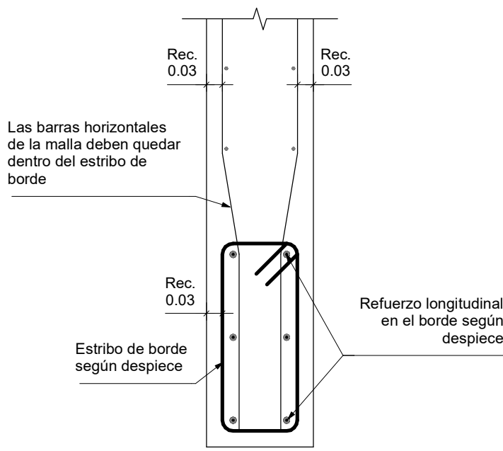
DETALLE ELEMENTO DE BORDE Escala 1 : 10
