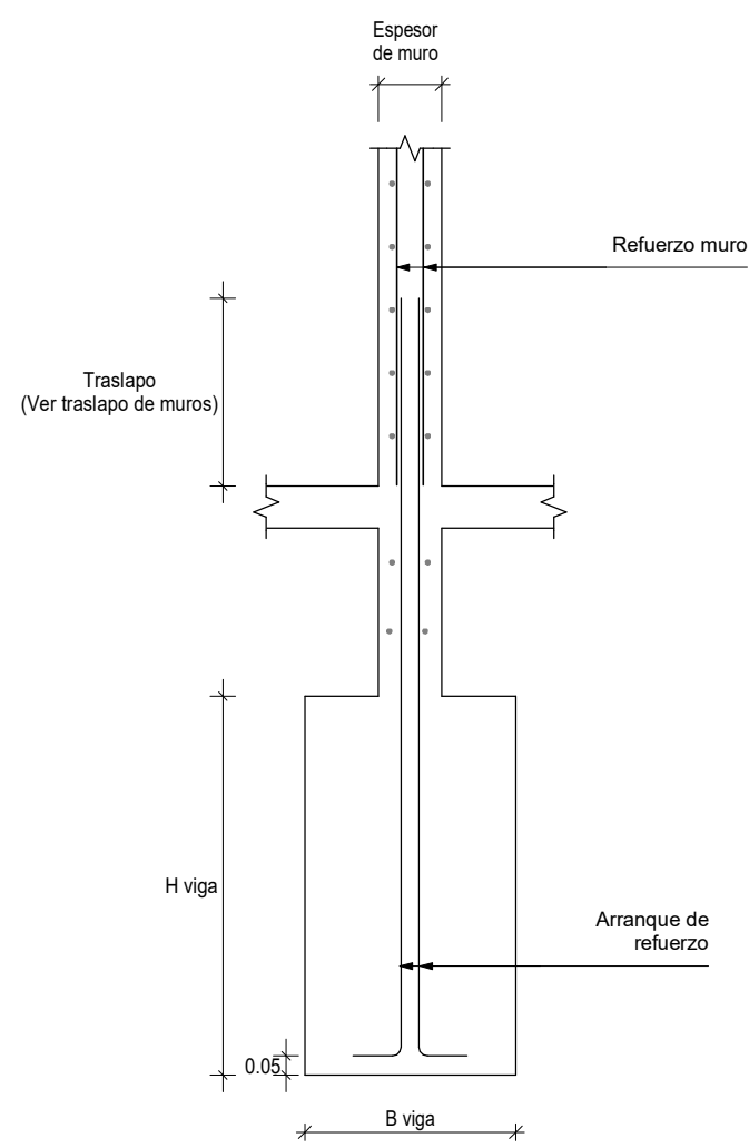
DETALLE ARRANQUE DE VARILLAS MUROS e≥0.15m Escala 1 : 20
