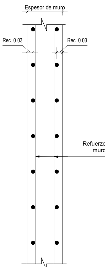
DETALLE RECUBRIMIENTO EN MUROS e≥0.15m
