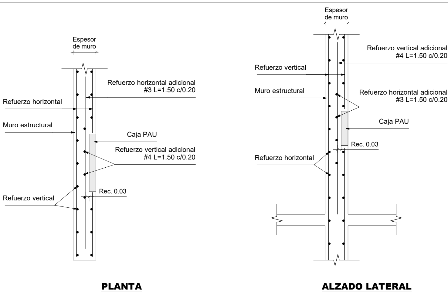
DETALLE REFUERZO ADICIONAL MUROS CON CAJAS PAU Escala 1 : 20
