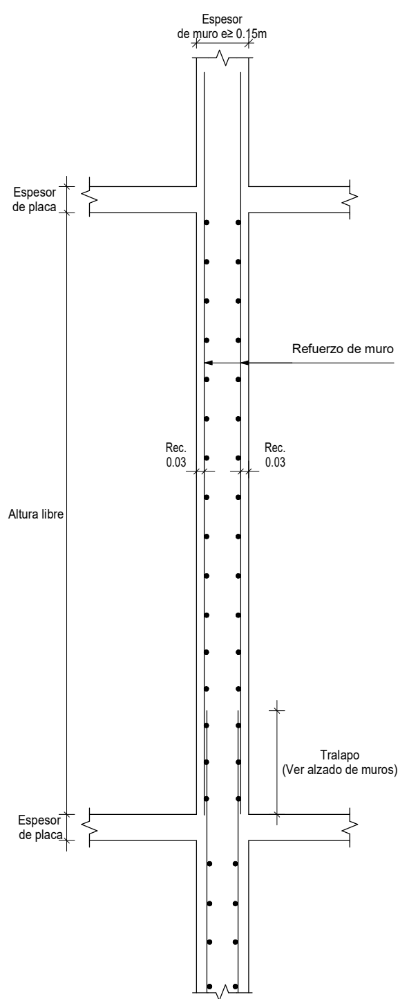
CORTE TRANSVERSAL MUROS e≥0.15m Escala 1 : 20
